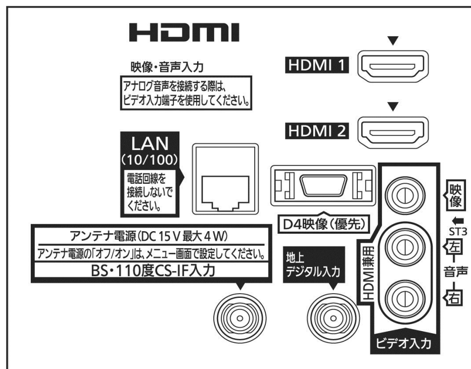
〈背面端子〉
